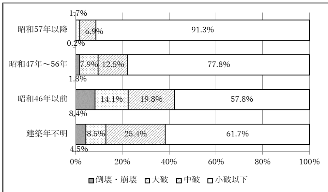
〔阪神・淡路大震災における建築物の被災状況（年代区分別）〕
